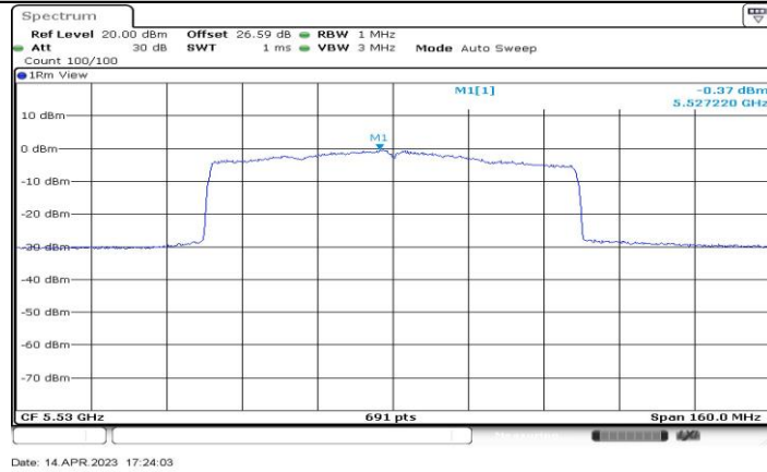
11BE80-CDD_Ant1_5530
