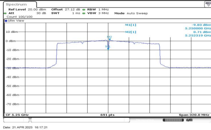
11AX160-CDD_Ant2_5250_UNII-2A
