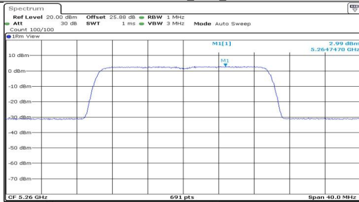
11BE20-CDD_Ant4_5240
