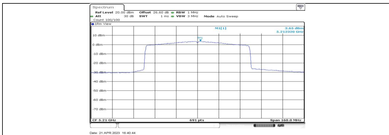
11BE80-CDD_Ant2_5210
