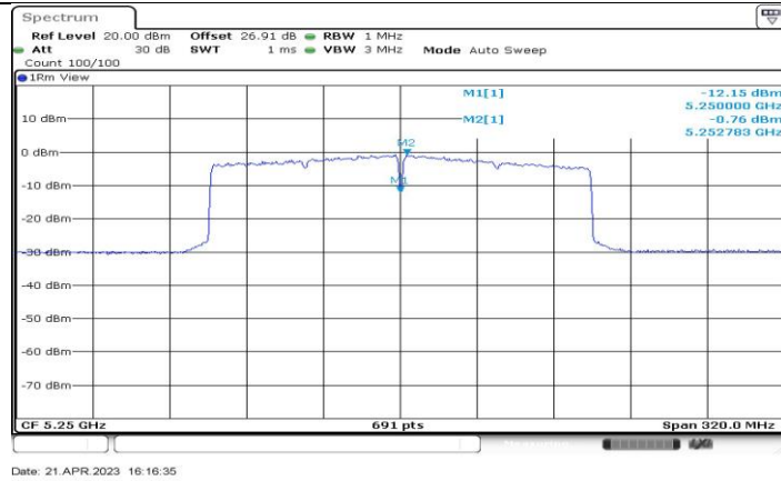
11AX160-CDD_Ant1_5250_UNII-2A
