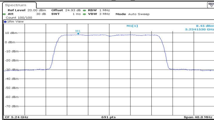
11BE20-CDD_Ant3_5240
