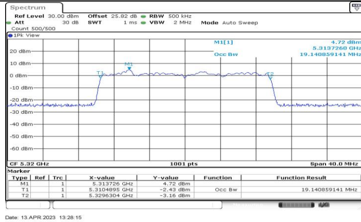
11BE20-CDD_Ant2_5320
