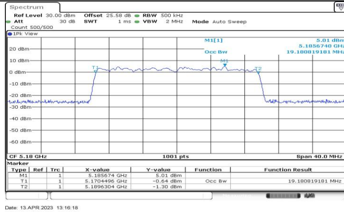
11BE20-CDD_Ant1_5180
