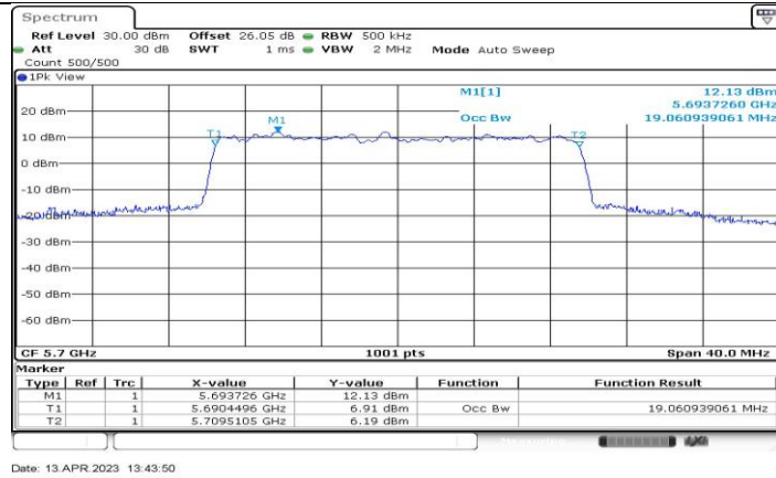
11BE20-CDD_Ant1_5700
