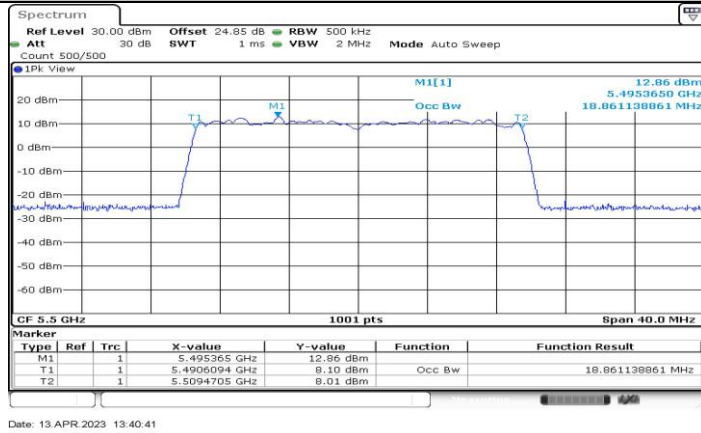
11BE20-CDD_Ant4_5500
