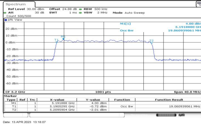
11BE20-CDD_Ant3_5200
