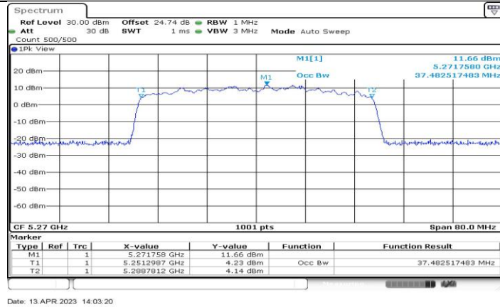
11BE40-CDD_Ant3_5270
