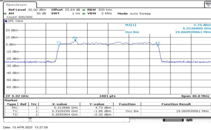
11BE20-CDD_Ant1_5320
