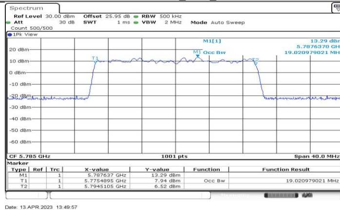
11BE20-CDD_Ant1_5785
