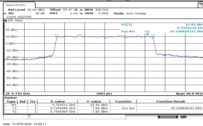
11BE20-CDD_Ant4_5745
