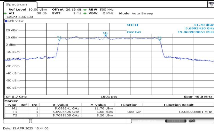
11BE20-CDD_Ant2_5700
