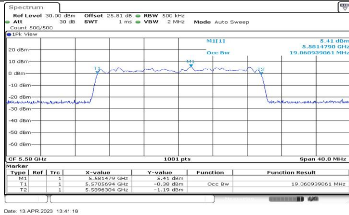
11BE20-CDD_Ant1_5580
