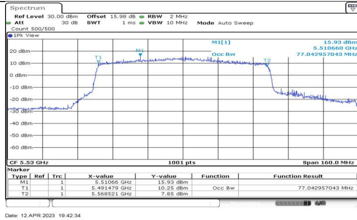
11AX80-CDD_Ant2_5530
