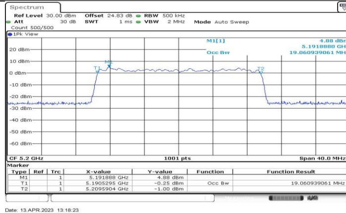
11BE20-CDD_Ant4_5200
