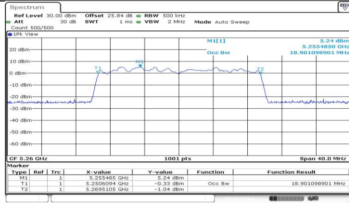
11BE20-CDD_Ant1_5260
