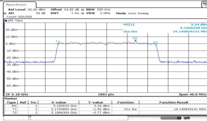
11BE20-CDD_Ant3_5180
