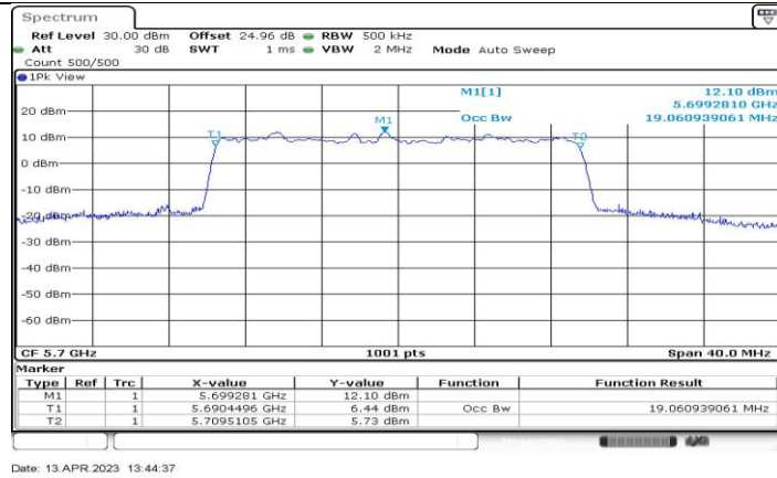
11BE20-CDD_Ant4_5700
