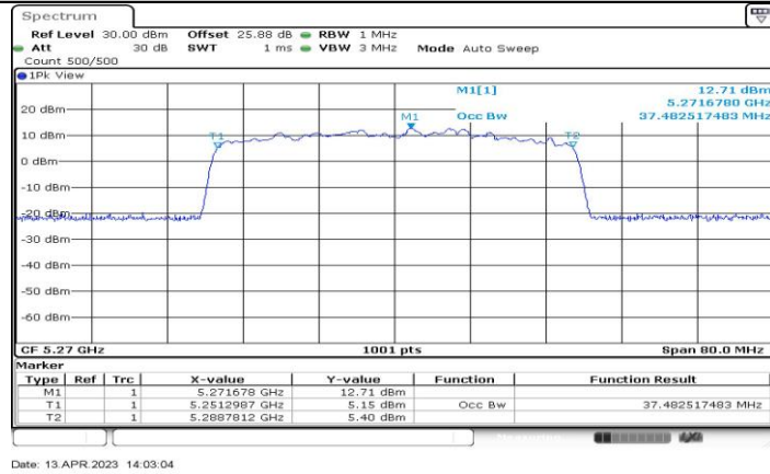
11BE40-CDD_Ant2_5270
