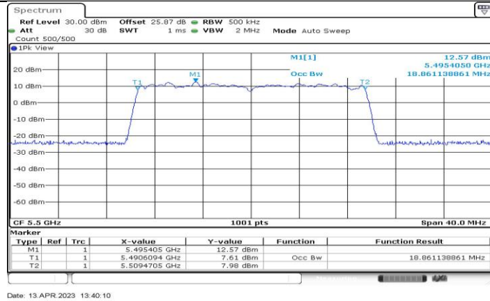
11BE20-CDD_Ant2_5500
