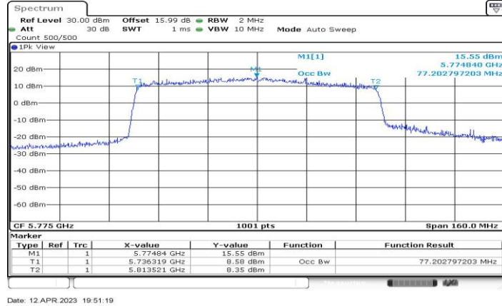
11AX80-CDD_Ant2_5775
