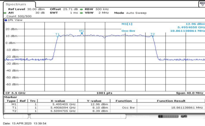
11BE20-CDD_Ant1_5500
