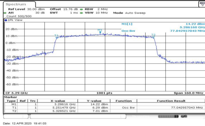
11AX80-CDD_Ant1_5290
