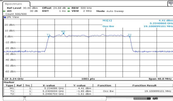
11BE20-CDD_Ant4_5240
