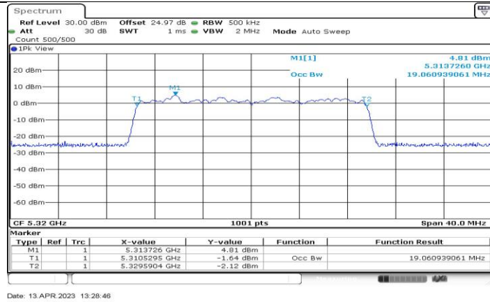
11BE20-CDD_Ant4_5320
