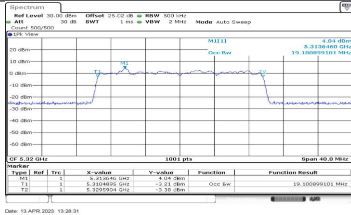
11BE20-CDD_Ant3_5320
