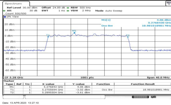
11BE20-CDD_Ant3_5280
