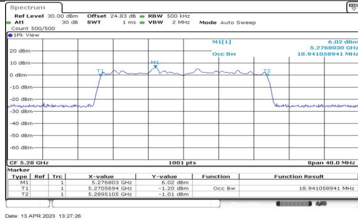
11BE20-CDD_Ant4_5280
