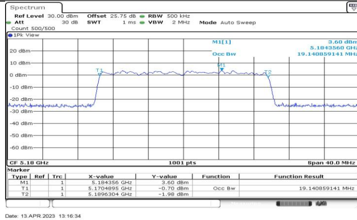
11BE20-CDD_Ant2_5180
