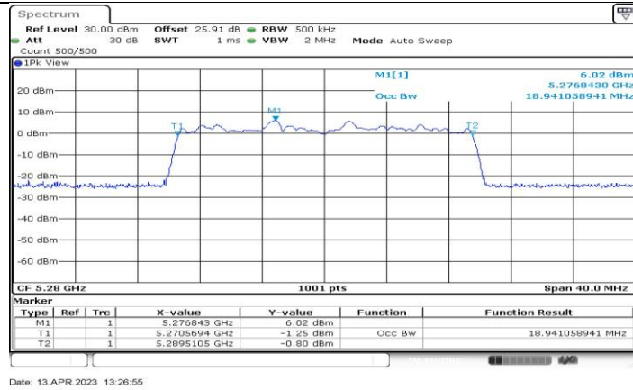
11BE20-CDD_Ant2_5280
