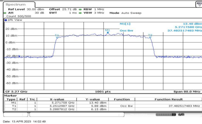
11BE40-CDD_Ant1_5270
