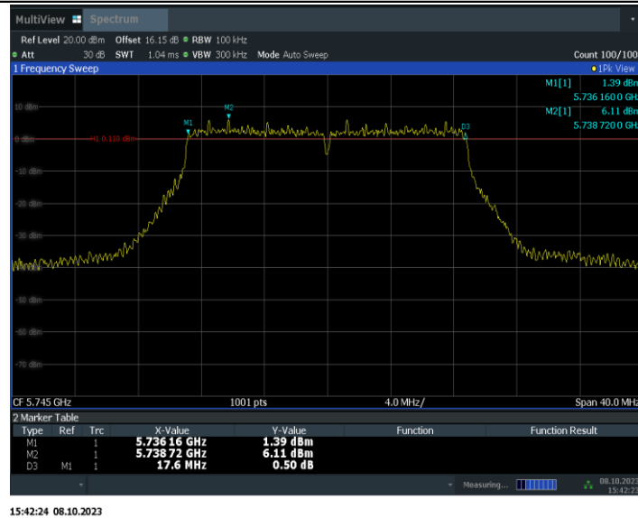
11AC20MIMO_Ant15_5745
