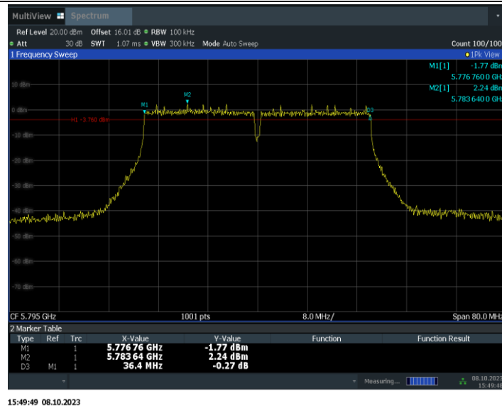
11AC80MIMO_Ant9_5775
