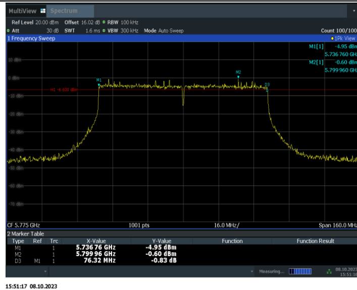
11AC80MIMO_Ant15_5775
