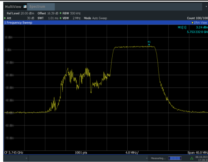
11AX20MIMO_Ant9_5745_106Tone_RU54
