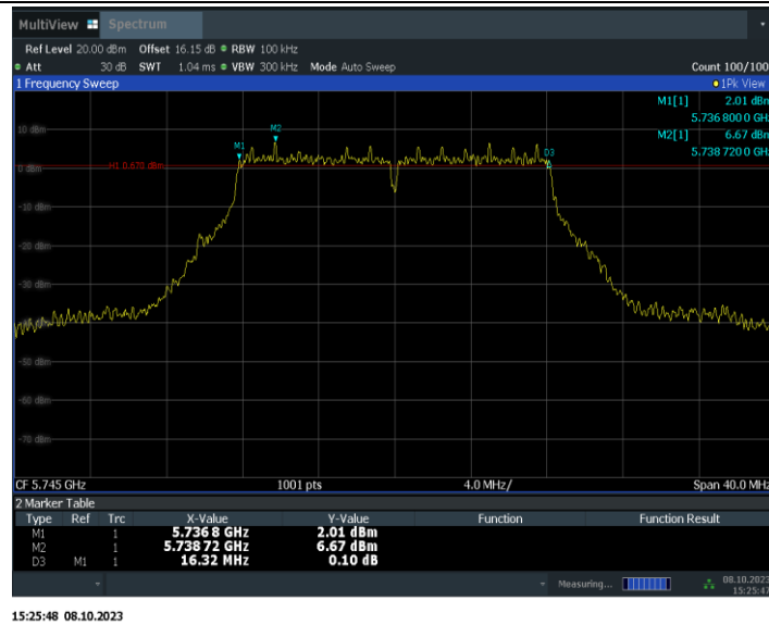
11A-MIMO_Ant15_5745
