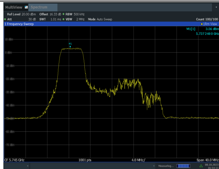
11AX20MIMO_Ant15_5745_52Tone_RU37
