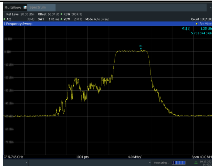
11BE20MIMO_Ant9_5745_52+26_OFDMA_3
