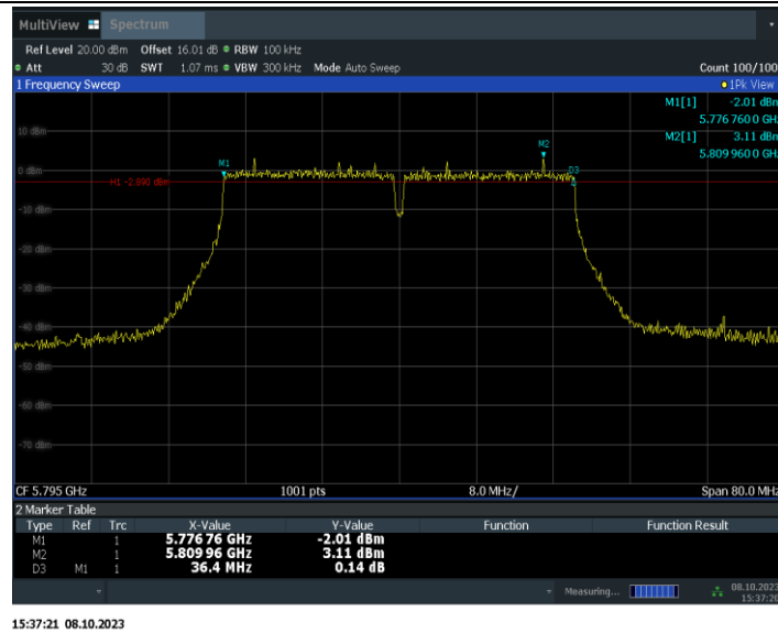
11AC20MIMO_Ant9_5745
