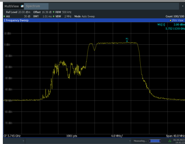
11BE20MIMO_Ant9_5745_106+26_OFDMA_2
