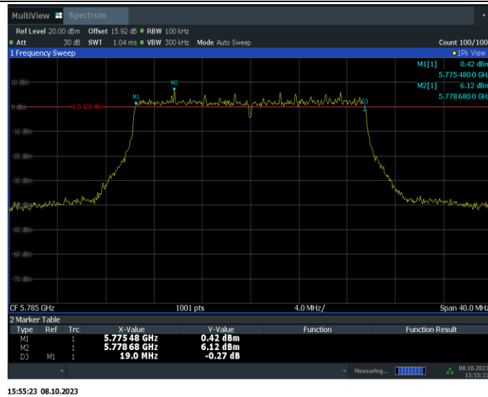
11AX20MIMO_Ant15_5785
