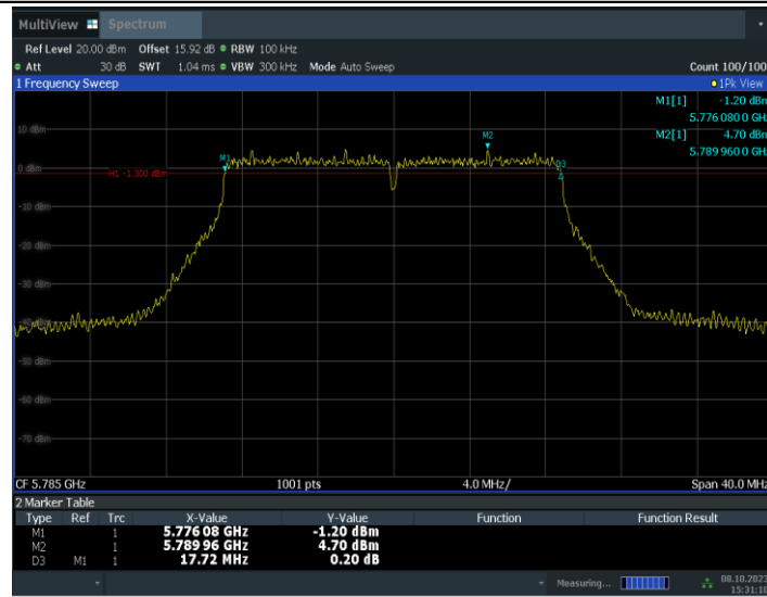
11N20MIMO_Ant9_5785
