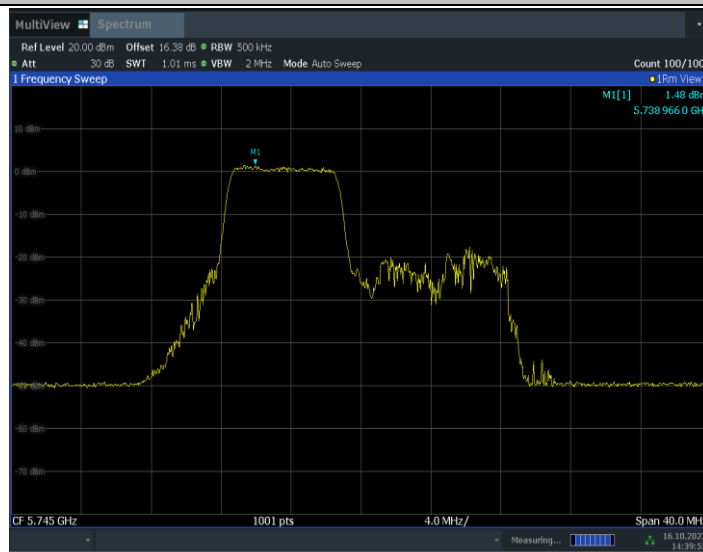
11BE20MIMO_Ant9_5745_52+26_OFDMA_1
