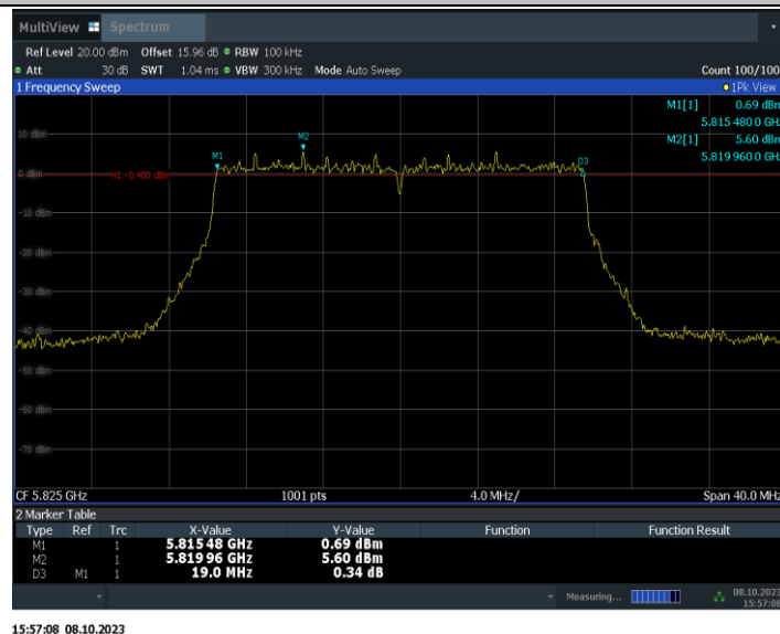
11AX20MIMO_Ant9_5825
