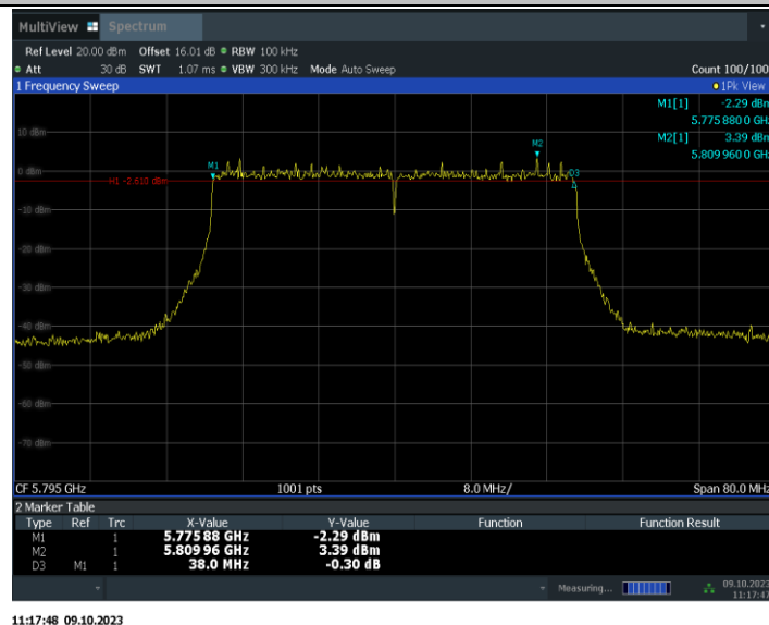
11AX40MIMO_Ant15_5795
