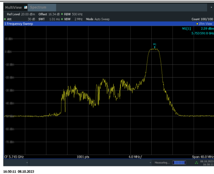
11AX20MIMO_Ant15_5745_52Tone_RU37
