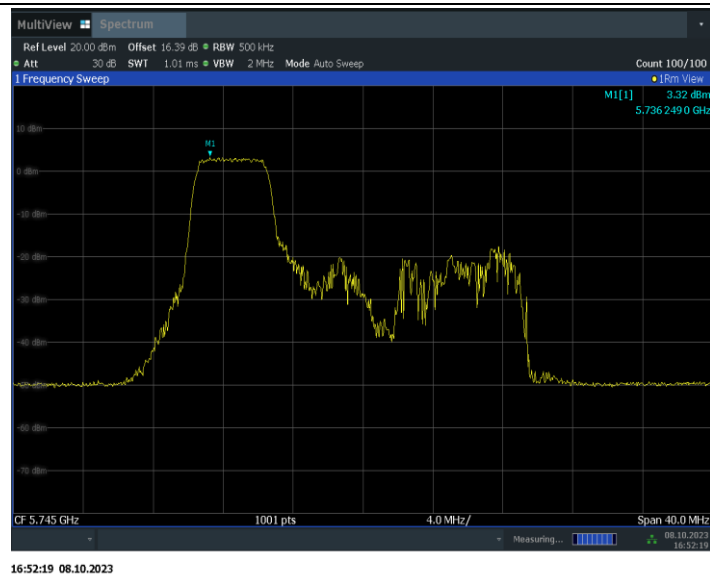
11AX20MIMO_Ant9_5745_52Tone_RU40
