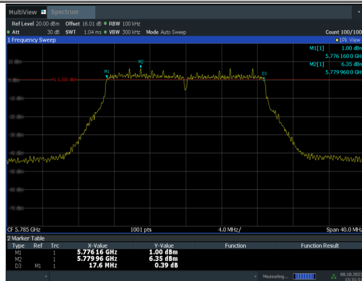
11N20MIMO_Ant15_5785
